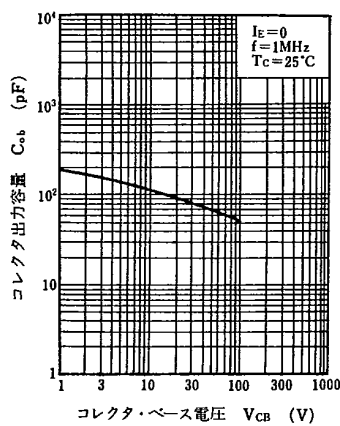
C_{ob} - V_{CB}
