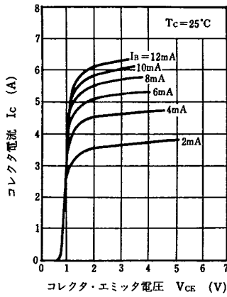
I_C - V_{CE}
