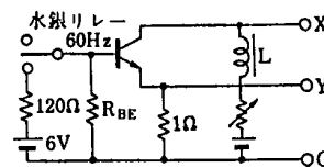
** E_{s/b} 測定回路 / E_{s/b} Test Circuit
