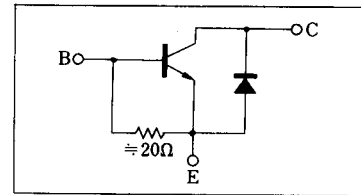
内部接続図 / Connection Diagram
