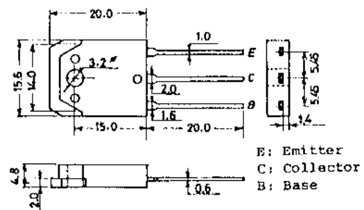
外形図 2022
