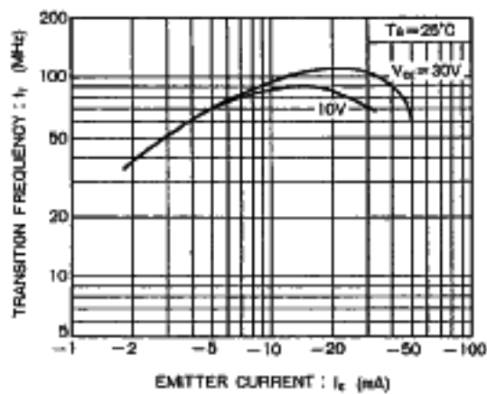
Fig.10 利得帯域積積—エミッタ電流特性
