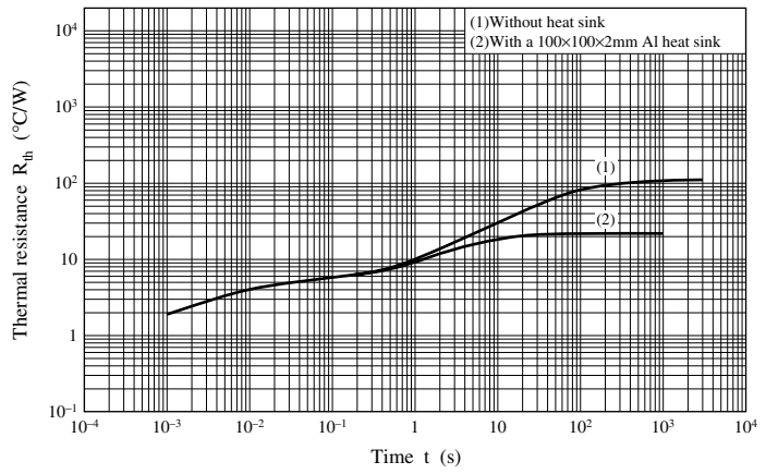
R_{th} - t
