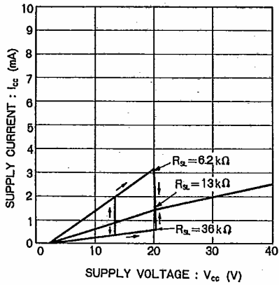
Fig. 5 消費電流—電源電圧特性
