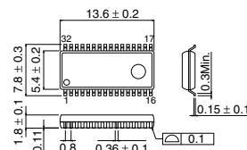
SSOP-A32
